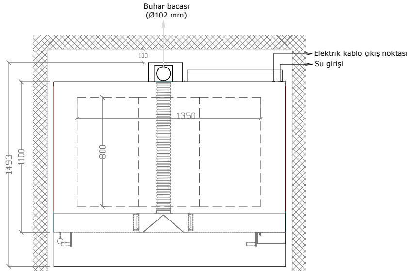
ÜST GÖRÜNÜS
