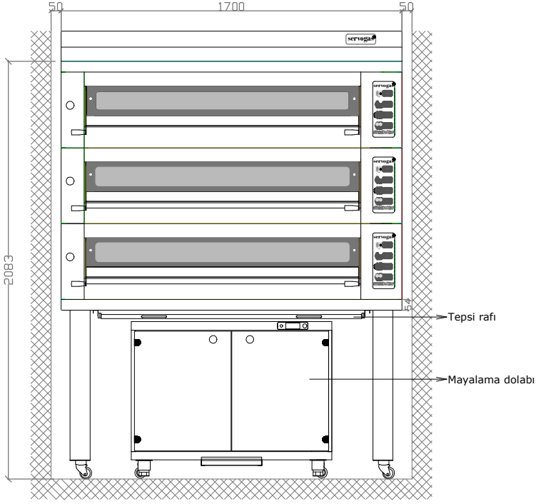
ÖN GÖRÜNÜS
