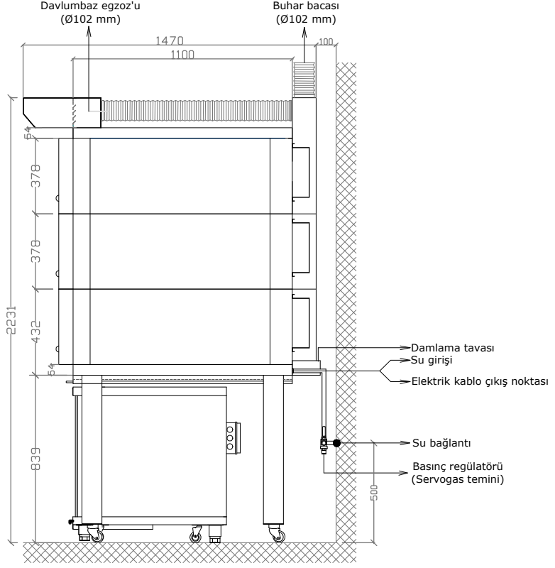
YAN GÖRÜNÜS
